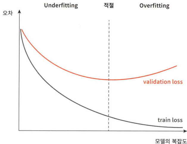
[그림 6-3] 모델 복잡도에 따른 오차 그래프
